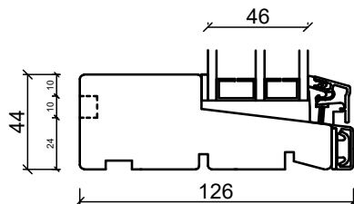
Bundkarm
