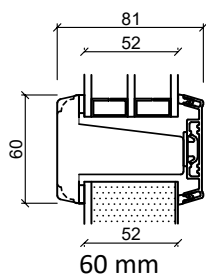
Vandret spændstykke
