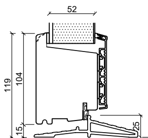
Glasfiber bundkarm
