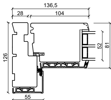
Vandret spændstykke
