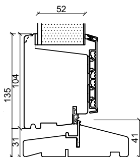
Hårdttræs bundkarm
