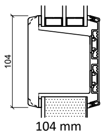
Glasfiber bundkarm
