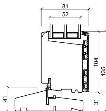
Hårdtræs bundkarm
