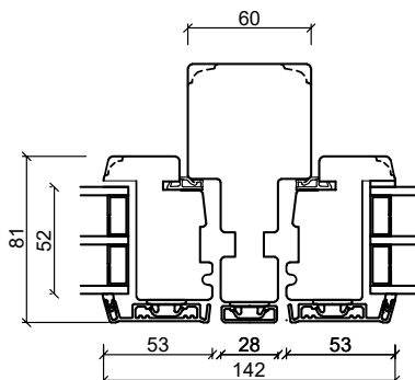
Lodpost
