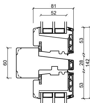
Tværpost – vandret
