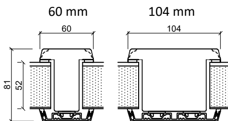
Lodret spændstykke
