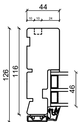
Sidekarm
