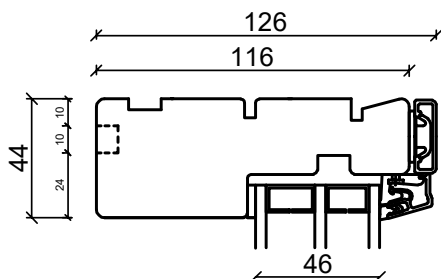
Overkarm
