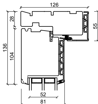
Lodret spændstykke
