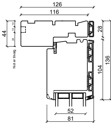
Overkarm
