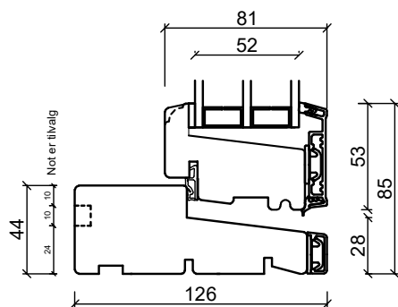
Bundkarm
