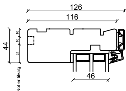
Sidekarm
