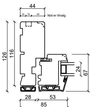
Sidekarm
