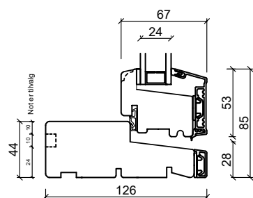
Bundkarm
