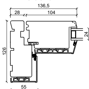
Lodret spændestykke
