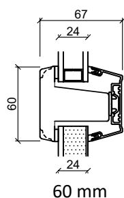
Vandret spændestykke
