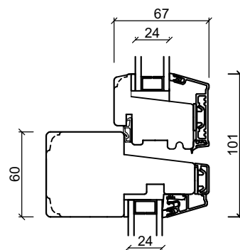
Tværpost
