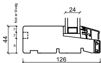
Bundkarm
