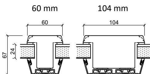
Lodret spændestykke
