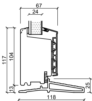
Glasfiber bundkarm
