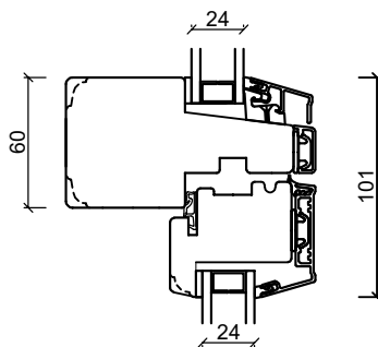
Tværpost
