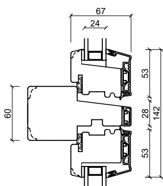
Tværpost – vandret
