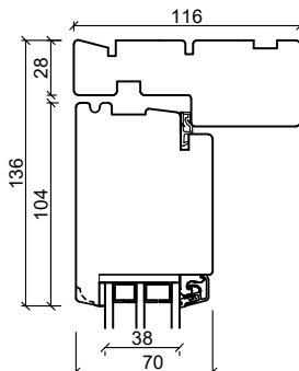
Lodret spændestykke
