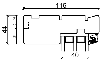
Overkarm
