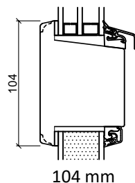
Glasfiber bundkarm
