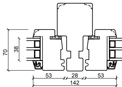
Lodpost
