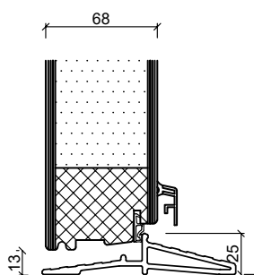
Glasfiber bundkarm
