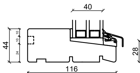
Bundkarm
