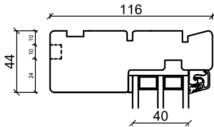
Overkarm
