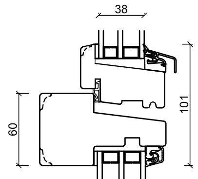
Tværpost
