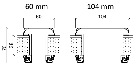
Lodret spændestykke
