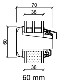
Vandret spændestykke
