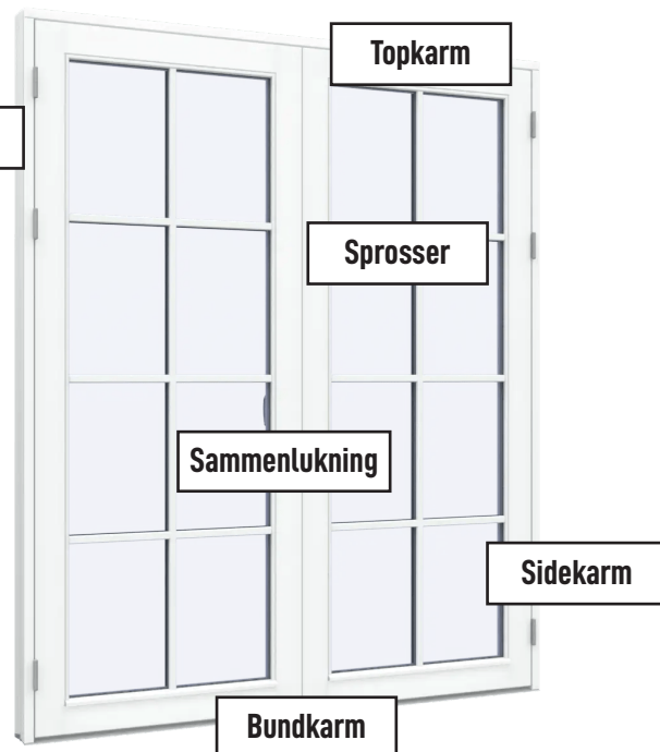
Hårdtræs bundkarm
