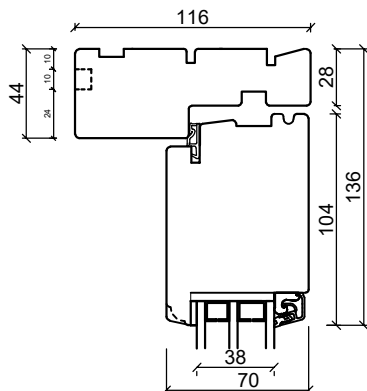
Overkarm
