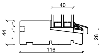
Bundkarm
