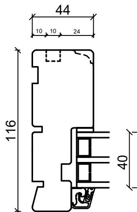
Bundkarm
