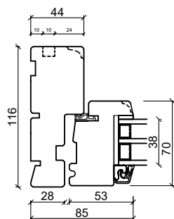
Sidekarm
