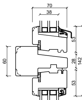
Tværpost – vandret
