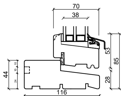
Bundkarm
