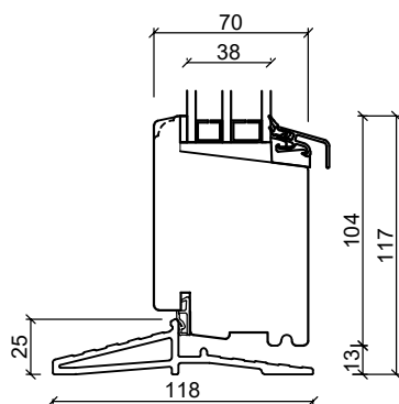
Glasfiber bundkarm
