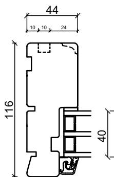
Sidekarm
