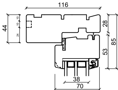
Overkarm
