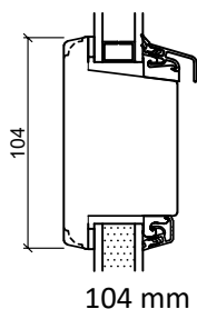
Glasfiber bundkarm
