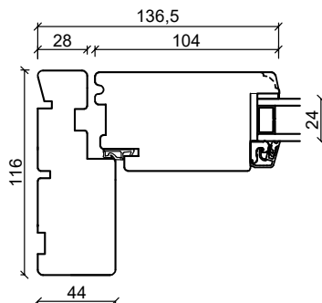
Lodret spændestykke
