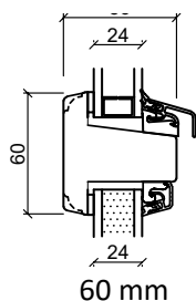
Vandret spændestykke
