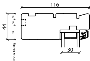
Overkarm
