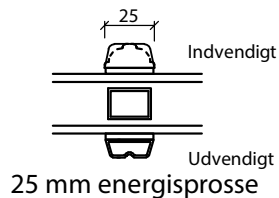
Energisprosse
