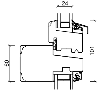
Tværpost
