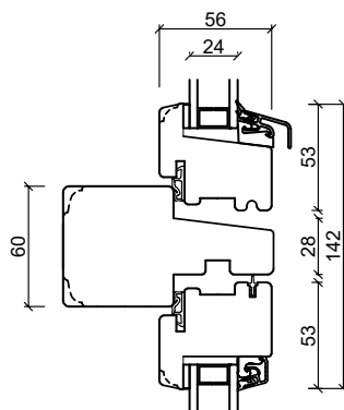
Tværpost – vandret
