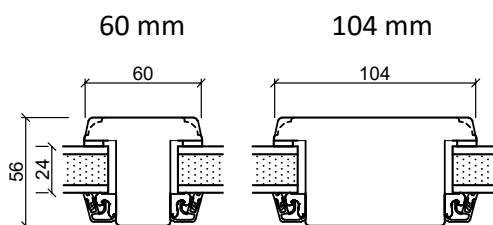
Lodret spændestykke
