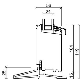
Glasfiber bundkarm
