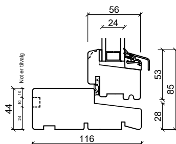
Bundkarm
