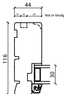
Sidekarm
