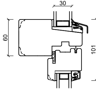
Tværpost
