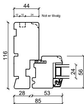
Sidekarm
