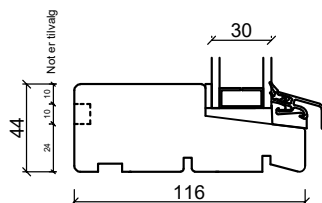
Bundkarm
