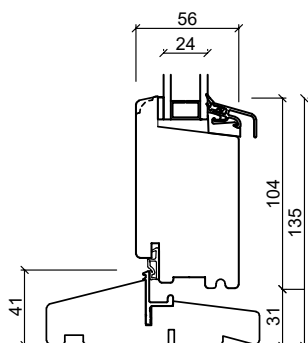
Hårdttræs bundkarm
