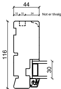
Sidekarm
