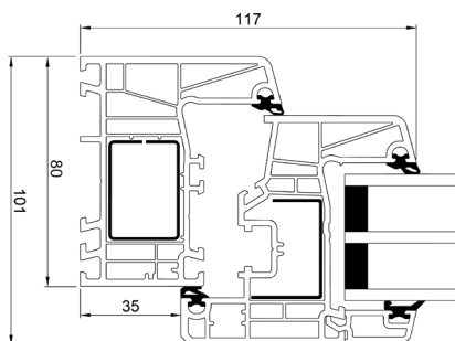
Sidekarm
