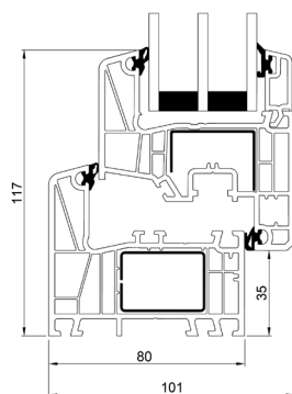
Bundkarm
