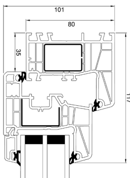
Overkarm
