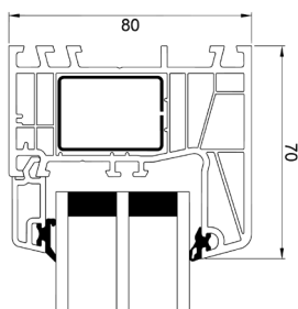
Overkarm
