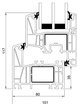
PVC bundkarm
