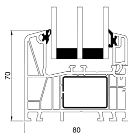
Bundkarm
