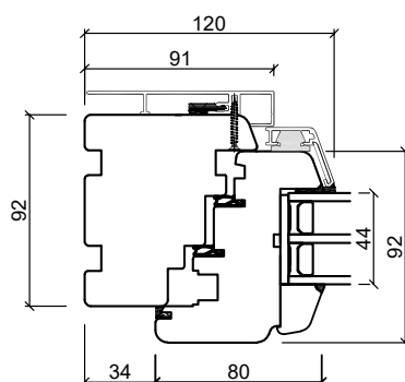
Hårdttræs bundkarm
