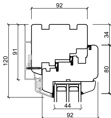
Tværpost - vandret
