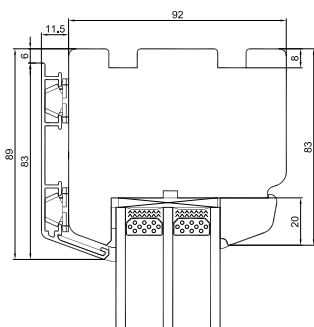
Overkarm
