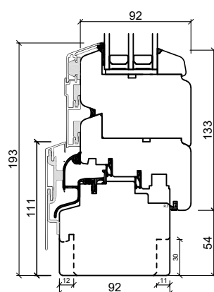
Hårdttræs bundkarm
