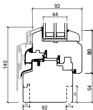
Bundkarm
