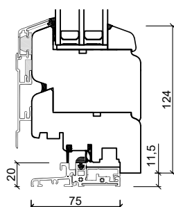
Alu bundkarm
