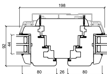
Tværpost
