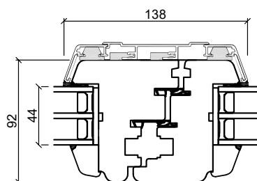
Midt dobbeltdør
