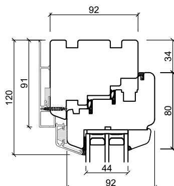
Midt dobbeltdør
