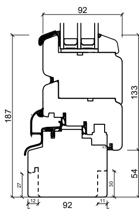
Hårdttræs bundkarm
