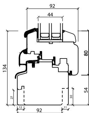
Sidekarm
