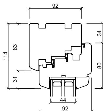
Overkarm
