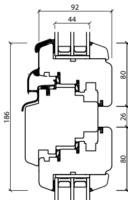
Tværpost - vandret
