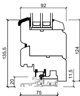
Alu bundkarm
