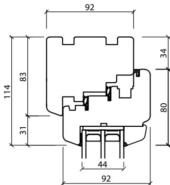
Tværpost - vandret
