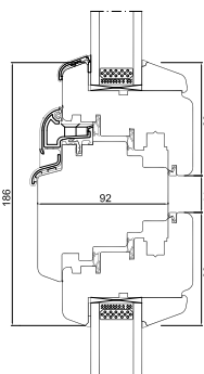
Tværpost – vandret
