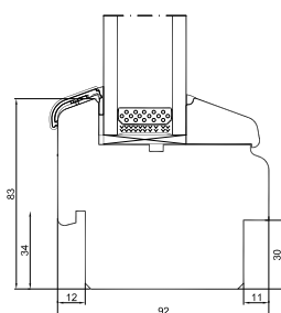
Bundkarm
