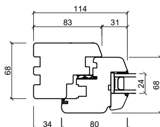
Sidekarm
