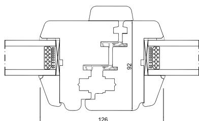
Midt dobbeltdør
