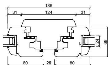
Tværpost
