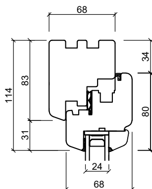
Tværpost
