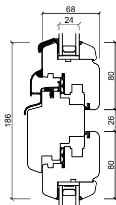
Tværpost – vandret
