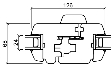
Midt dobbeltdør
