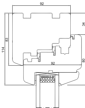
Tværpost
