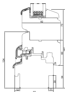
Hårdttræs bundkarm
