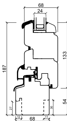
Hårdttræs bundkarm
