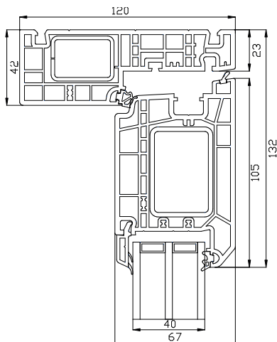
Overkarm
