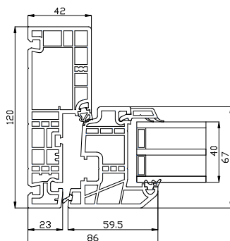
Sidekarm
