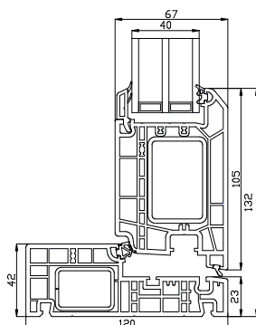
PVC bundkarm
