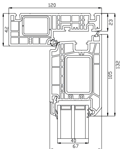
Sidekarm
