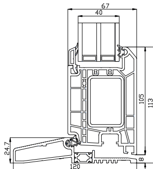
Alu bundkarm
