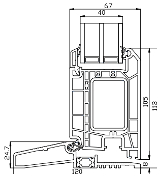
Alu bundkarm
