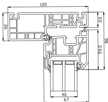
Overkarm
