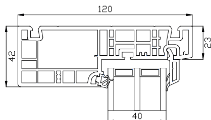
Overkarm
