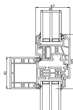
Tværpost
