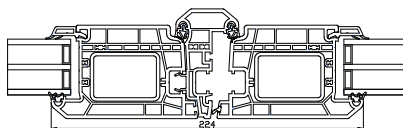
Sammenlukning
