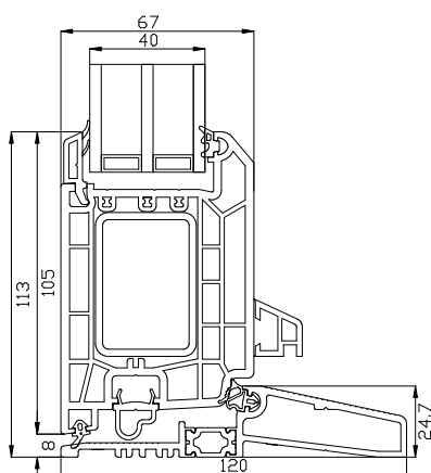
Bundkarm
