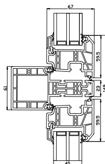
Tværpost – vandret
