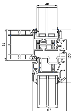
Tværpost
