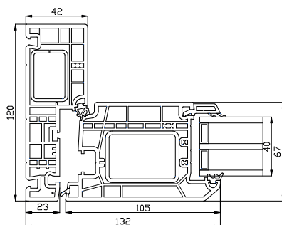
Sidekarm
