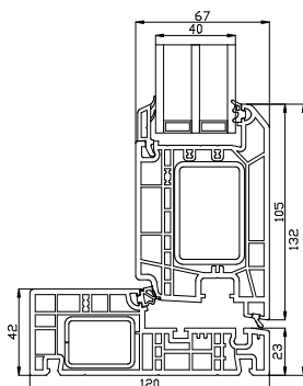
PVC bundkarm
