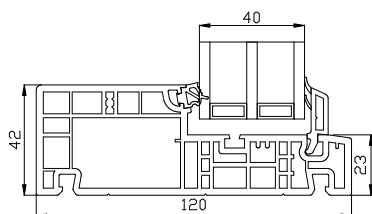
Bundkarm
