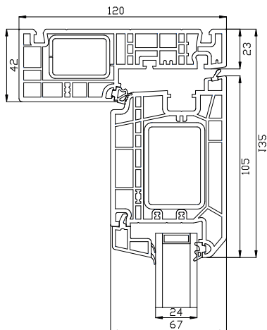
Overkarm
