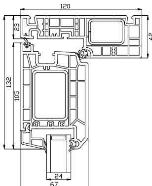
Overkarm
