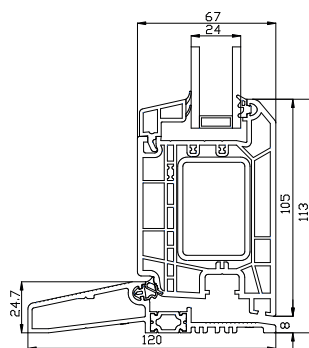
Alu bundkarm
