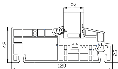
Bundkarm
