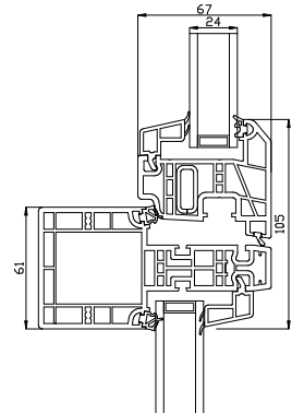
Tværpost
