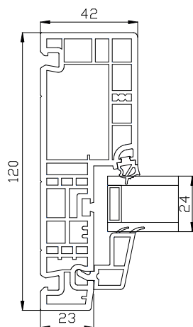
Bundkarm
