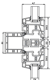
Tværpost – vandret
