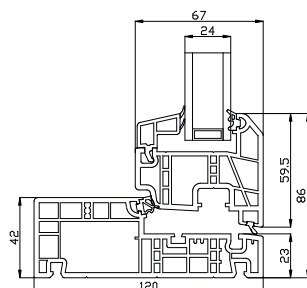
Bundkarm
