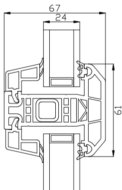
Spændestykke
