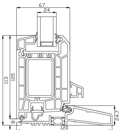
Bundkarm
