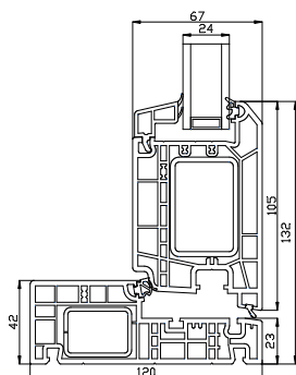
PVC bundkarm
