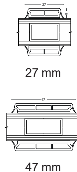
Energisprosse
