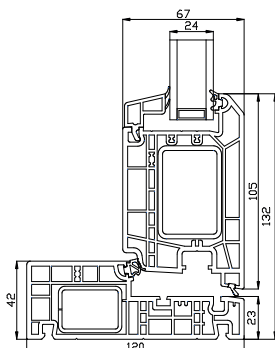
PVC bundkarm
