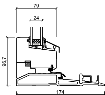
Bundkarm
