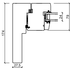
Sidekarm
