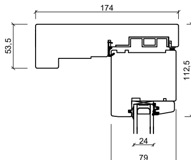
Overkarm
