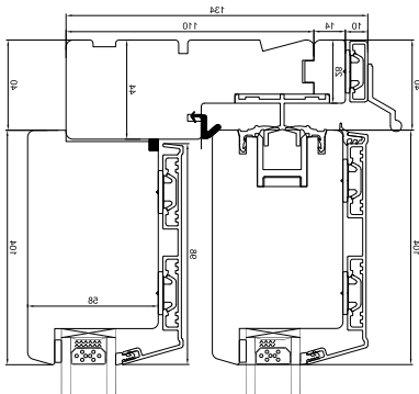
Overkarm
