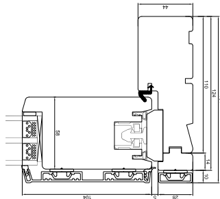
Sidekarm
