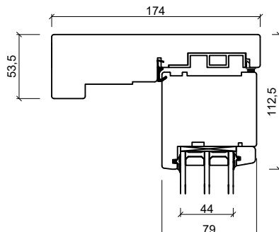
Sidekarm
