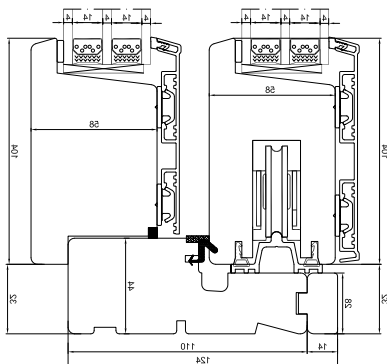
Bundkarm
