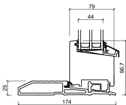
Bundkarm
