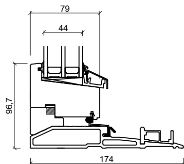
Bundkarm
