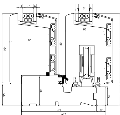
Bundkarm
