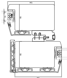
Midt hæveskydedør
