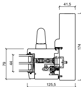
Sidekarm
