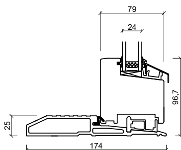
Bundkarm
