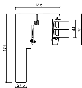
Bundkarm
