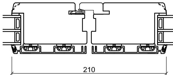
Sammenlukning
