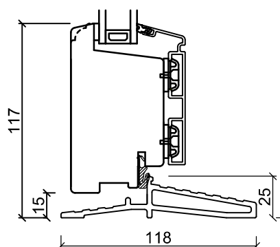
Glasfiber Bundkarm
