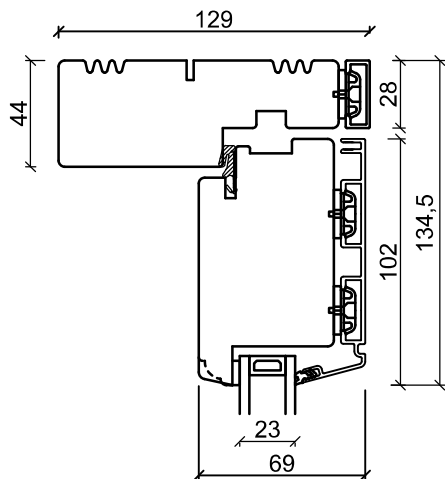
Overkarm
