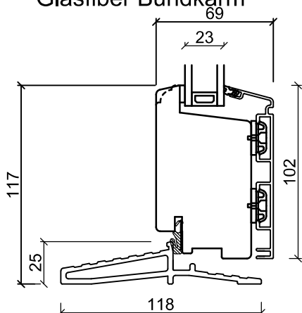
Glasfiber Bundkarm
