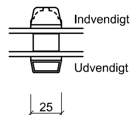
Energisprosse
