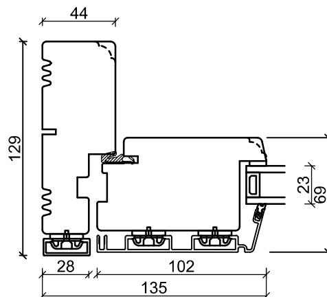
Sidekarm
