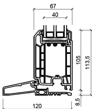
Bundkarm
