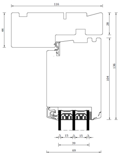
Overkarm
