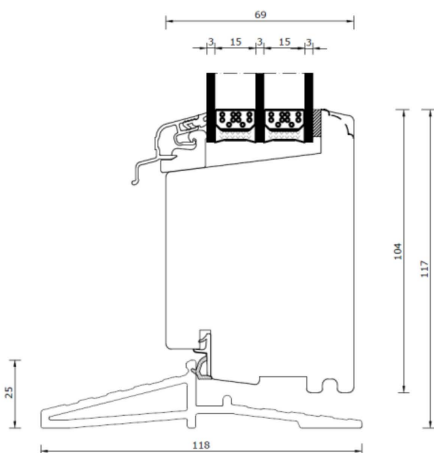
Glasfiber bundkarm
