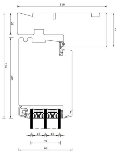
Hårdtræs Bundkarm
