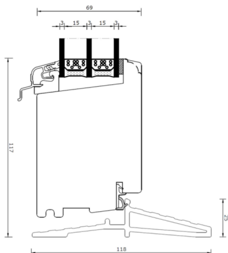
Glasfiber bundkarm
