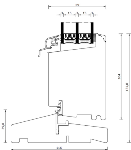
Glasfiber bundkarm
