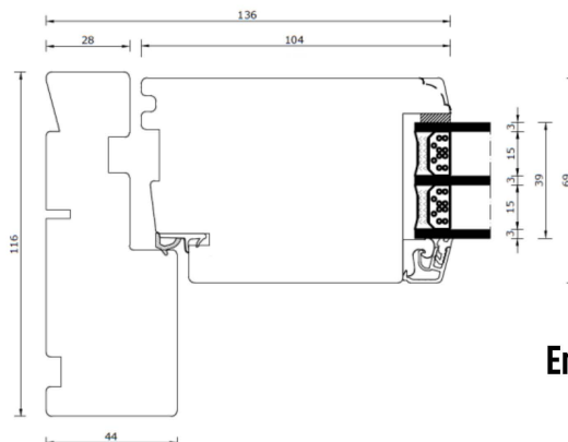
Sidekarm
