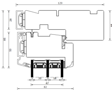
Overkarm
