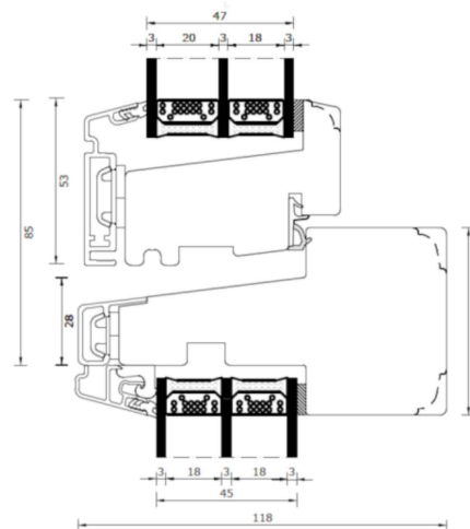
Vandret post
