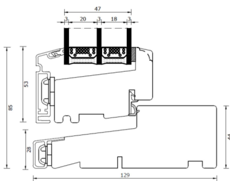
Bundkarm
