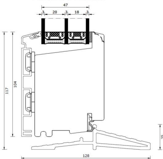
Glasfiber bundkarm
