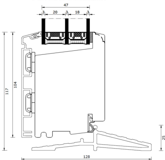
Glasfiber bundkarm
