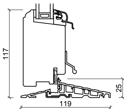
Alu-Bundkarm
