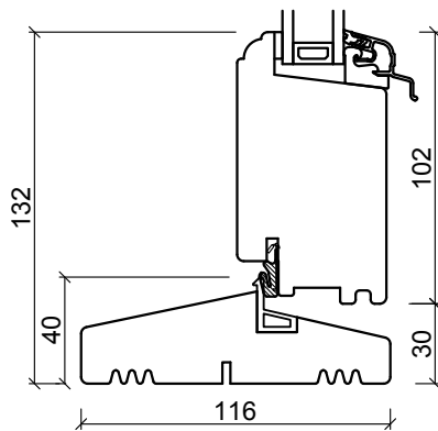
Hårdtræs-Bundkarm
