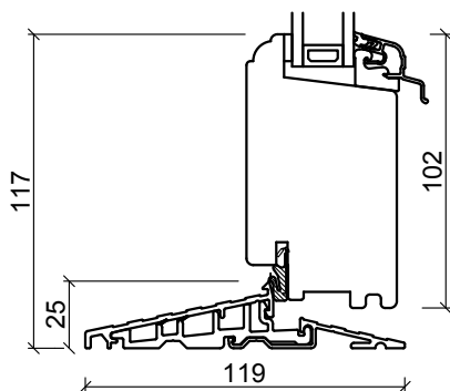
Alu-Bundkarm
