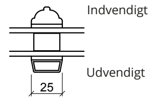
Energisprosser
