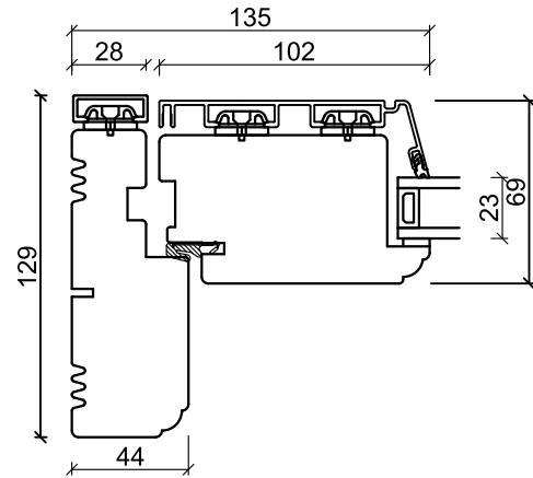
Sidekarm
