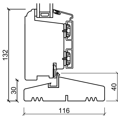
Hårdtræs Bundkarm
