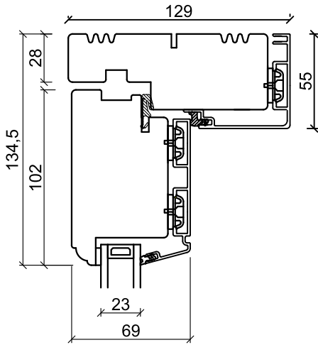
Overkarm
