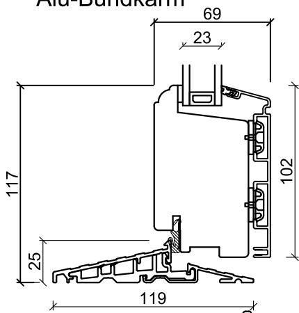
Alu-Bundkarm
