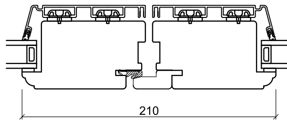
Sammenlukning
