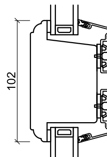
Spændestykke
