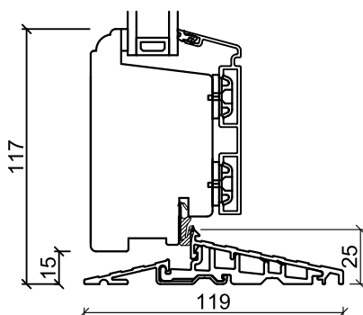
Alu-Bundkarm
