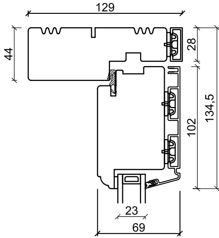
Overkarm
